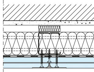
■ DC Profil 12 mm yalıtım şeridi ile
