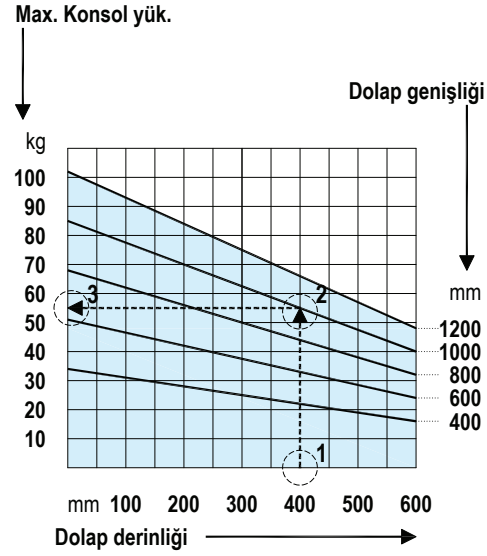
İzin verilen en fazla konsol yük (kg) - diagrama göre
