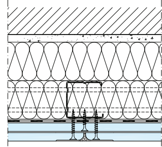
■ DC Profil 12 mm yalıtım şeridi ile
