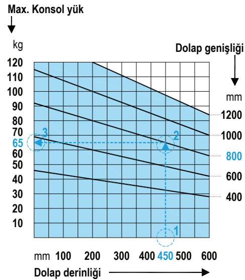
İzin verilen en fazla konsol yük (kg) - digrama göre
